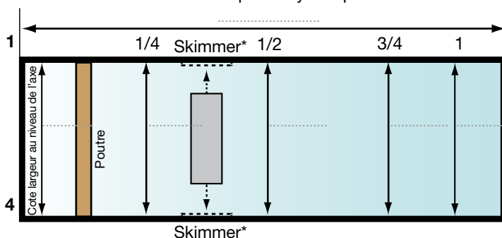
Dimensions de la piscine y compris la fosse
